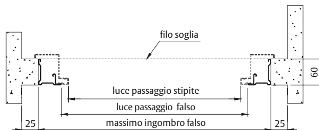
SEZIONE ORIZZONTALE
