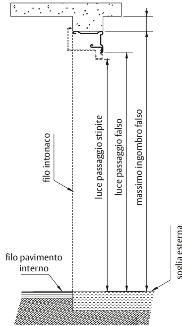
SEZIONE VERTICALE
